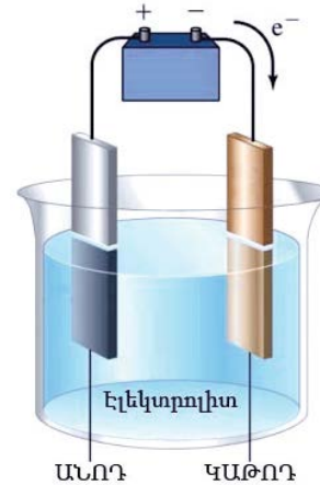
электролиз
