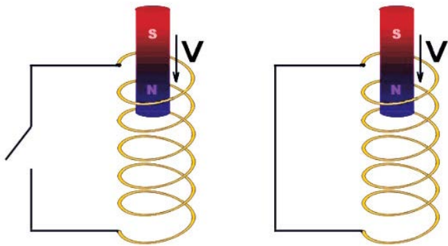
электромагнитная индукция
