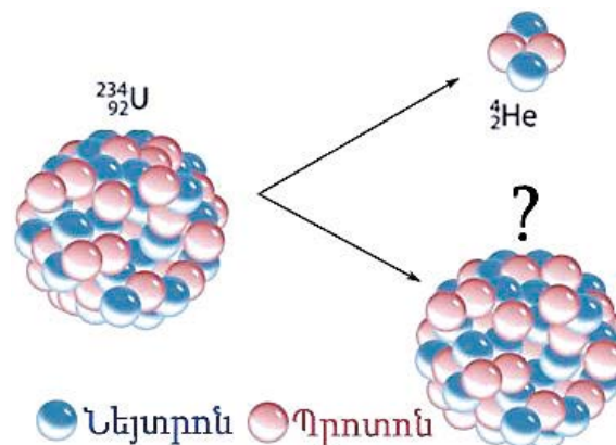
ядерный распад
